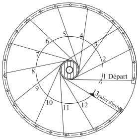
Escalier Colimaçon Ø1400 (avec limon)
