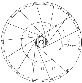
Escalier Colimaçon Ø1400 (sans limon)
